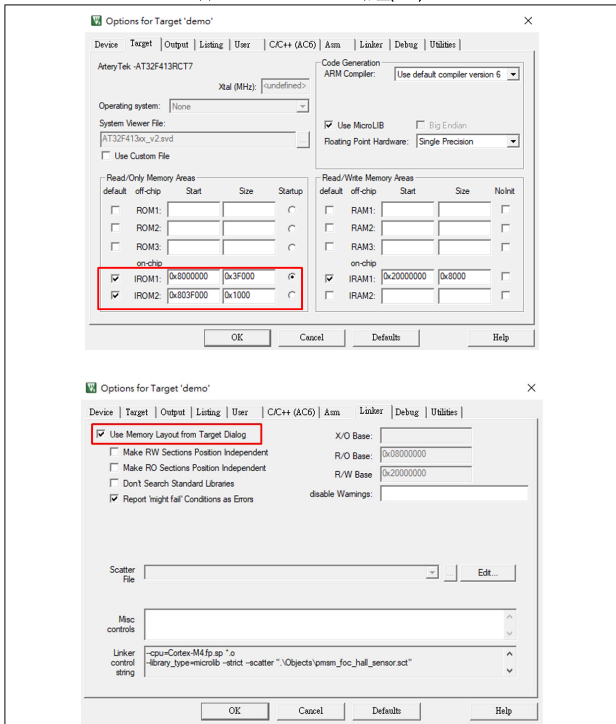
图 2. AT32F413RCT7 ROM 配置(Keil)
