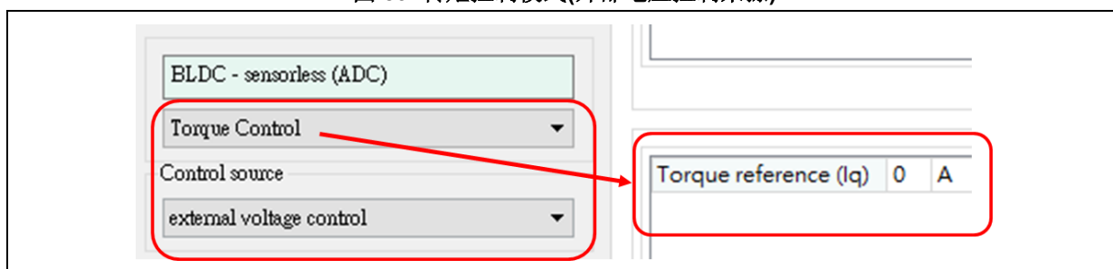
图 59 转矩控制模式(外部电压控制来源)
