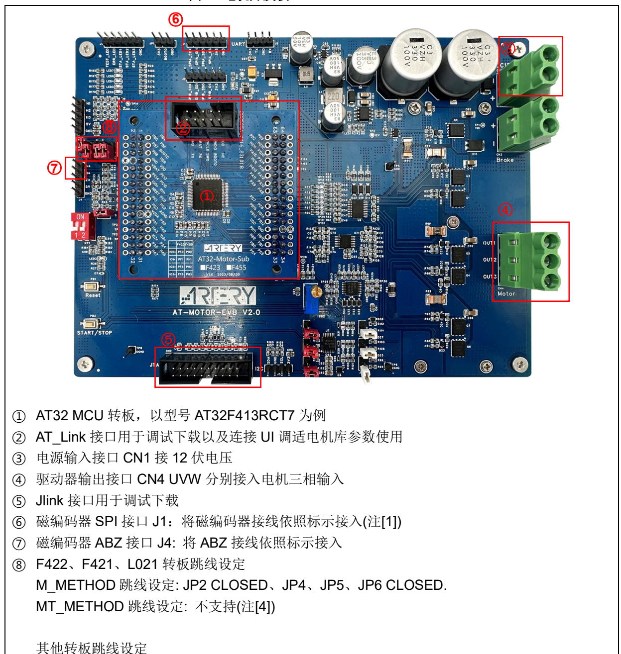
图 1. 电机开发板 AT-MOTOR-EVB V2.x
