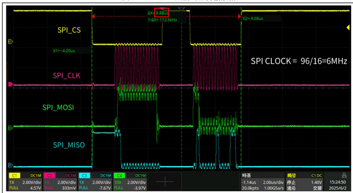
图 7. AS5047P 磁编码器传输数据
