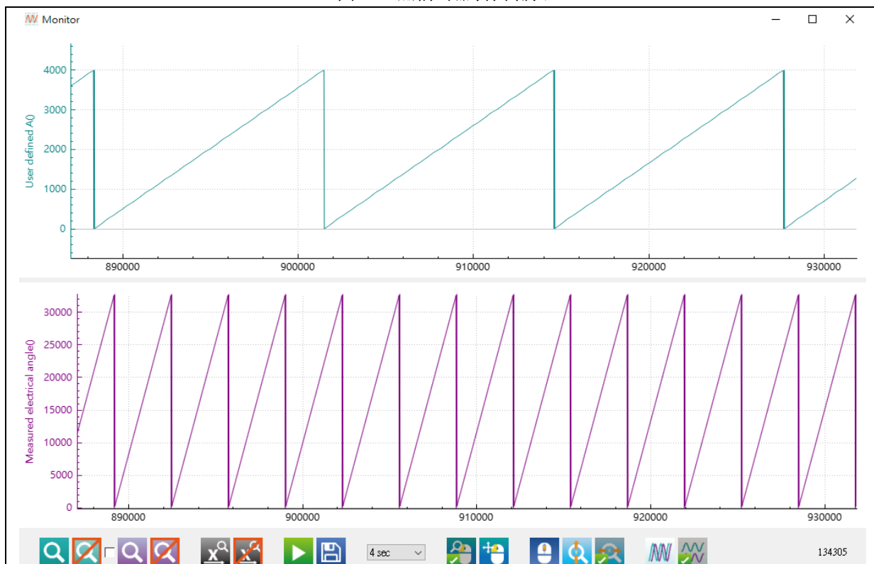
图 12. 磁编码器转向确认
