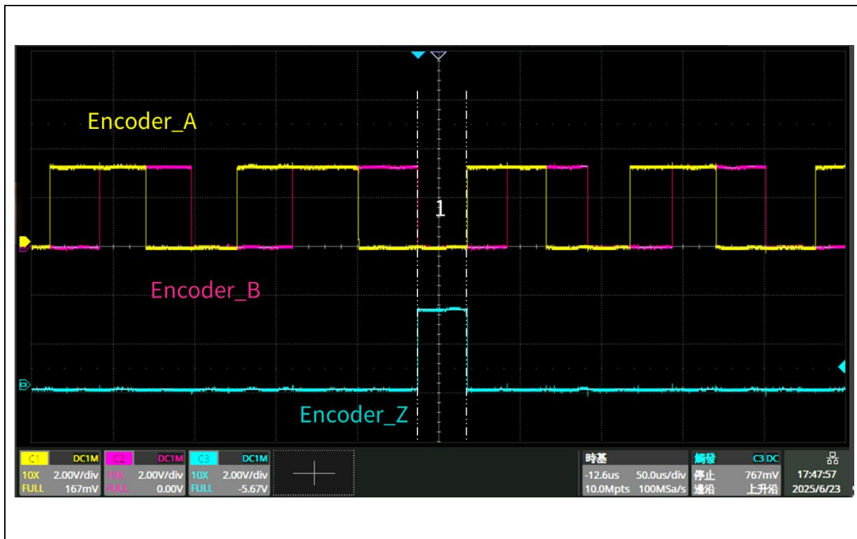
图 5. 磁编码器 ABZ 信号的关系图
